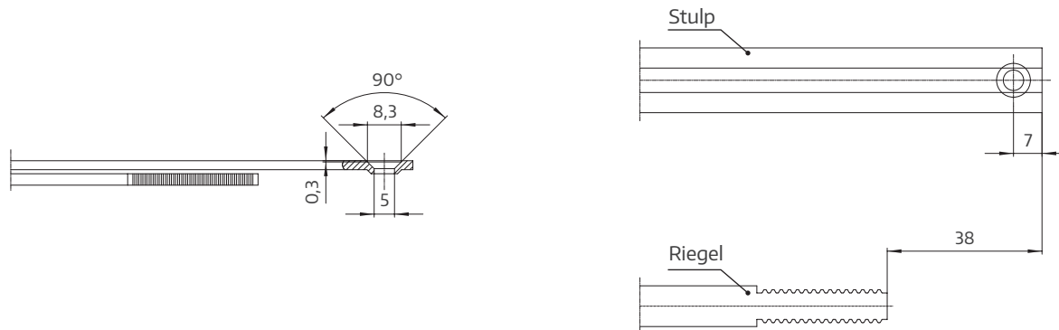
Abb. 1 - Stanzbild
