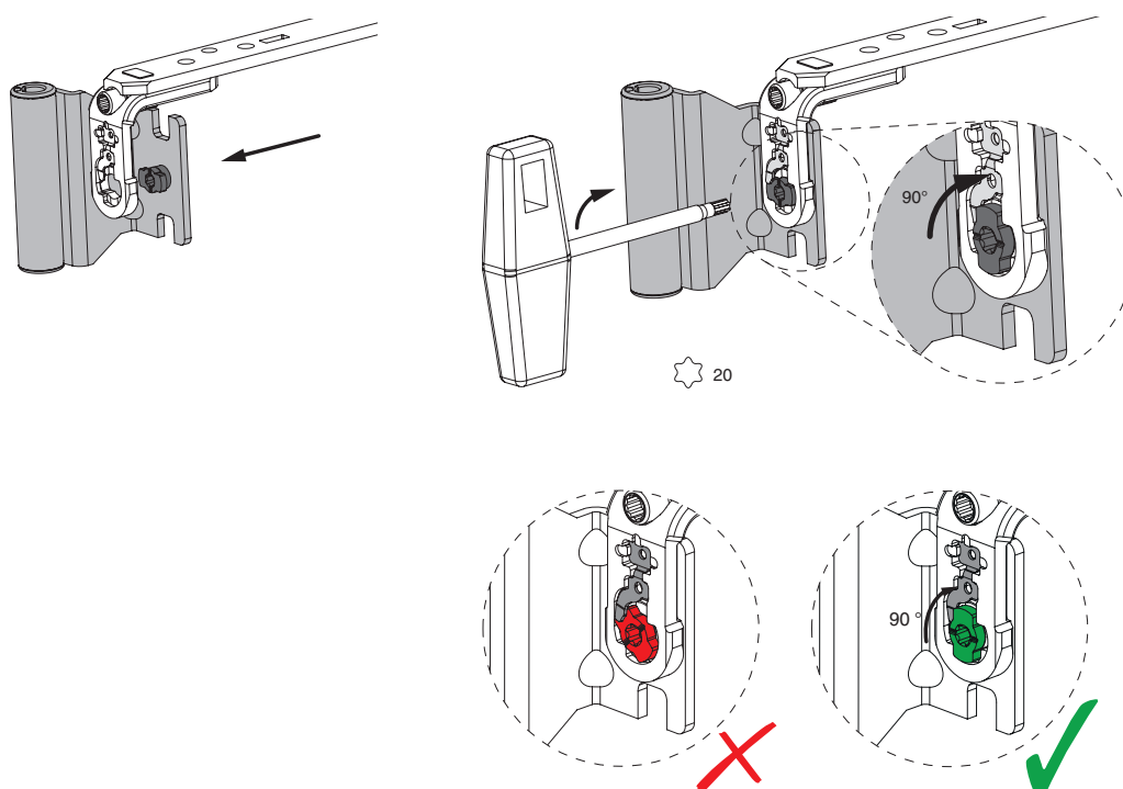
Abb. 2 - Bajonettverbindung
